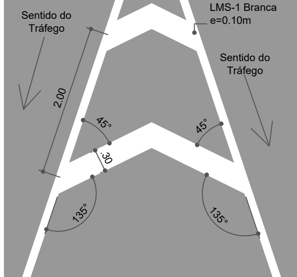
Marcação - Separação de fluxo de mesmo sentido ESC: 1:50
