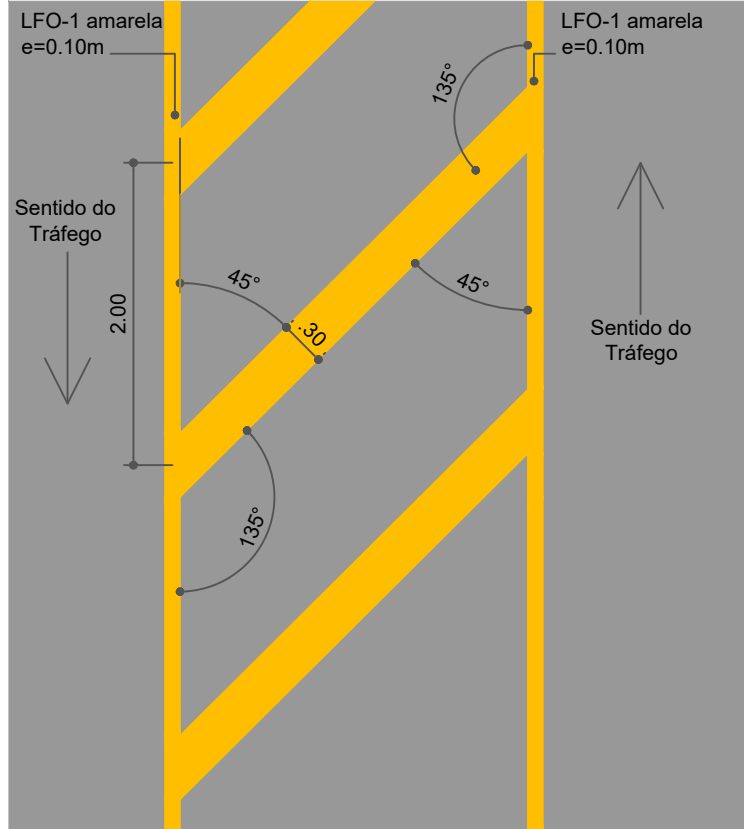
Marcação - Separação de fluxo de tráfego de sentido oposto ESC: 1:50
