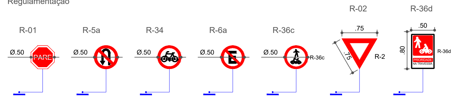
DET - Placas de Sinalização Vertical esc. 1:50
