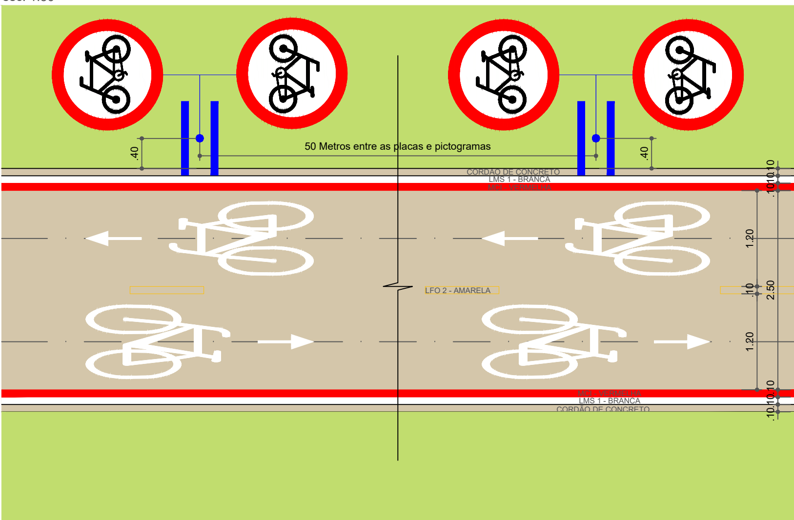
DET - Placas de Sinalização Vertical esc. 1:50
