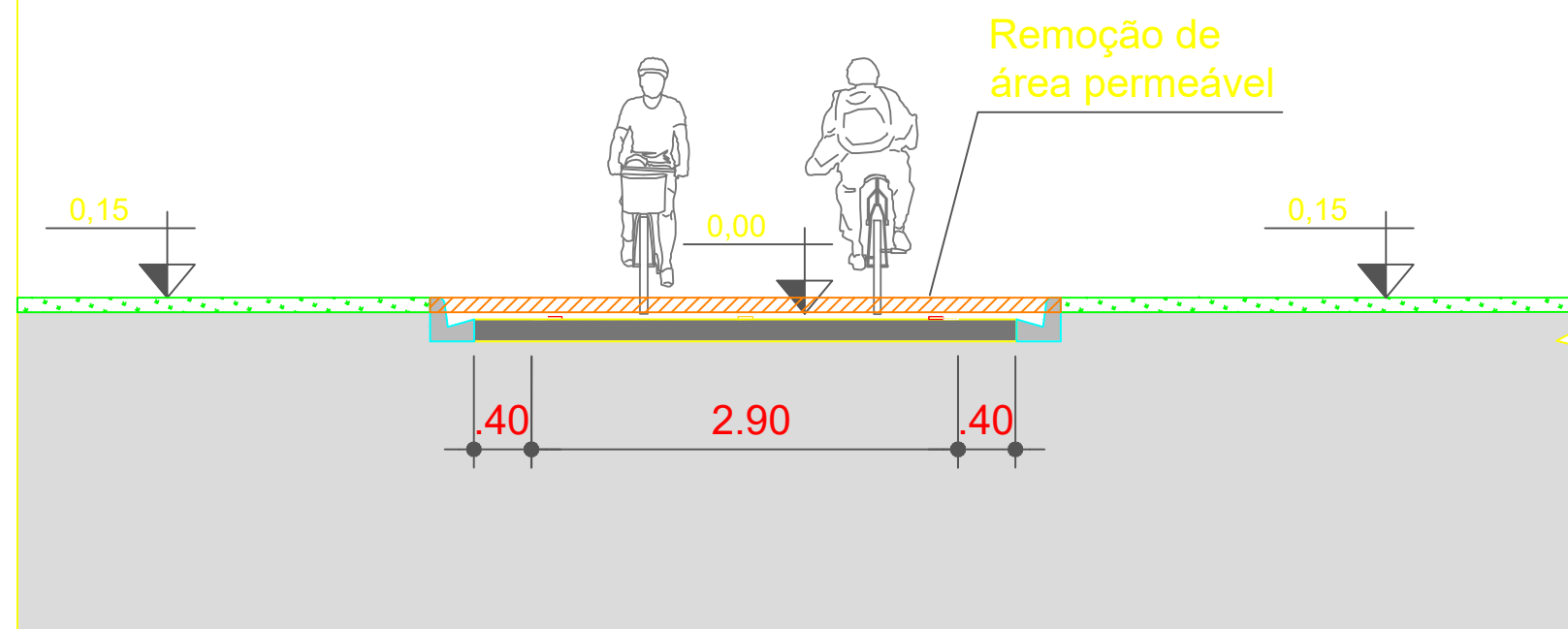
CORTE EE - ESC 1:50
