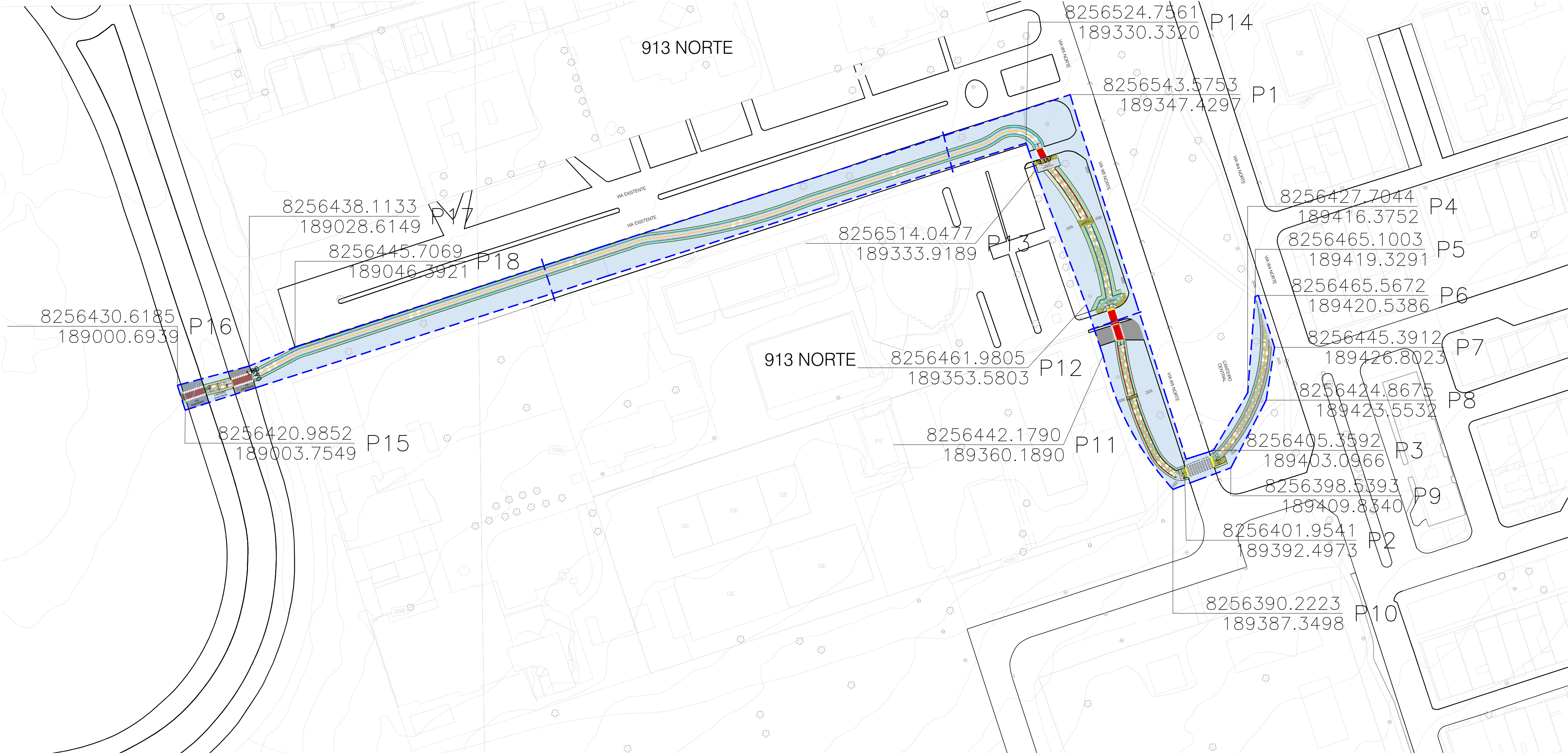
PLANTA GERAL ESCALA 1/250
