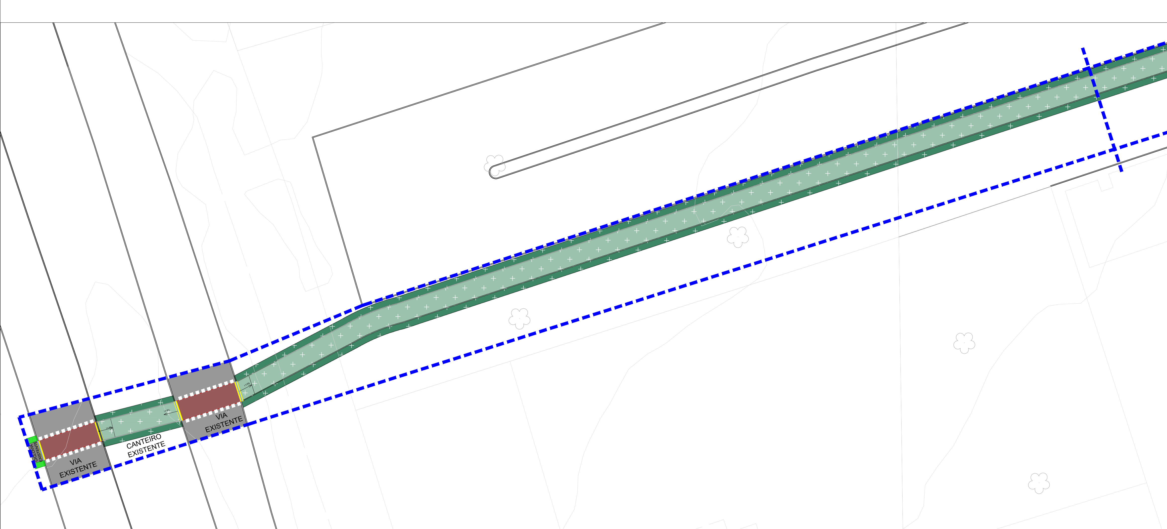
TRECHO 1 ESCALA 1/250
