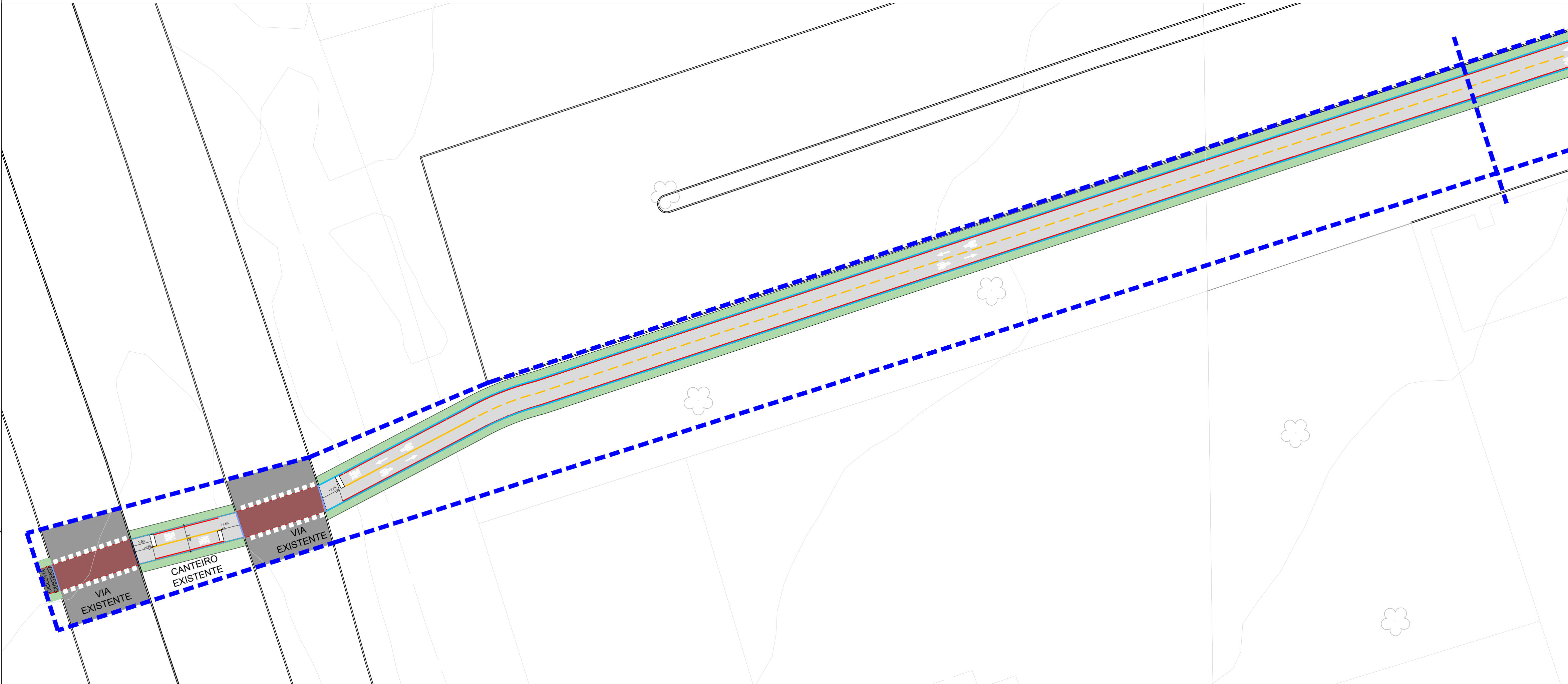
TRECHO 1 ESCALA 1/250
