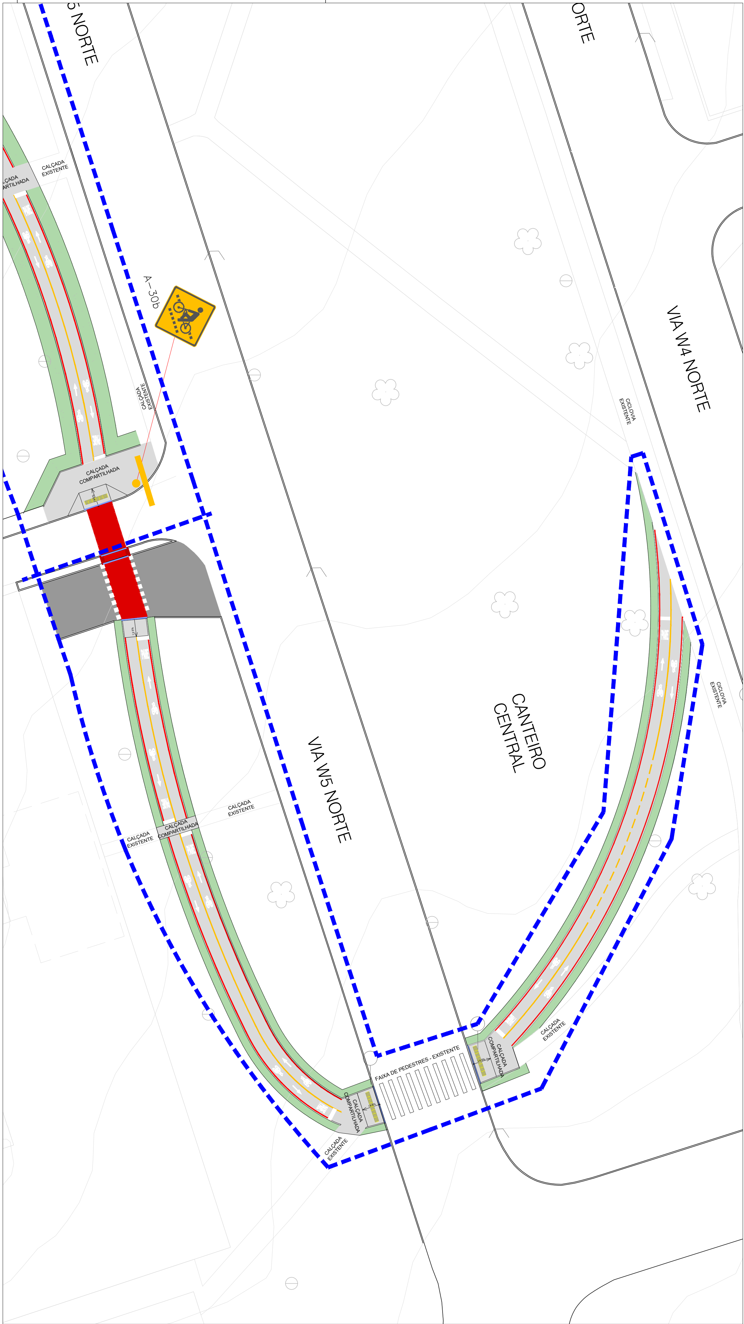
TRECHO 4 ESCALA 1/250
