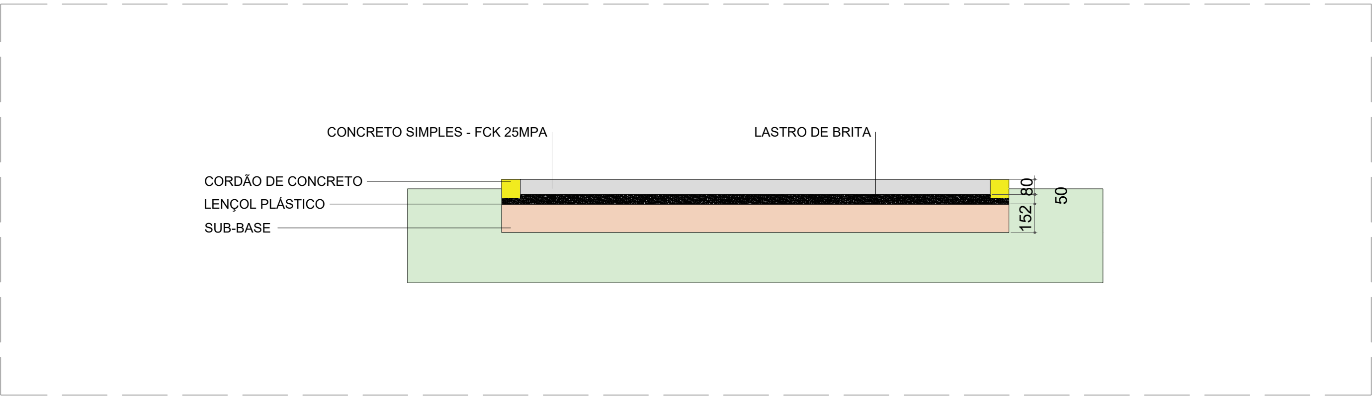
DETALHE 02 – CORTE DA CICLOVIA ESCALA 1/20
