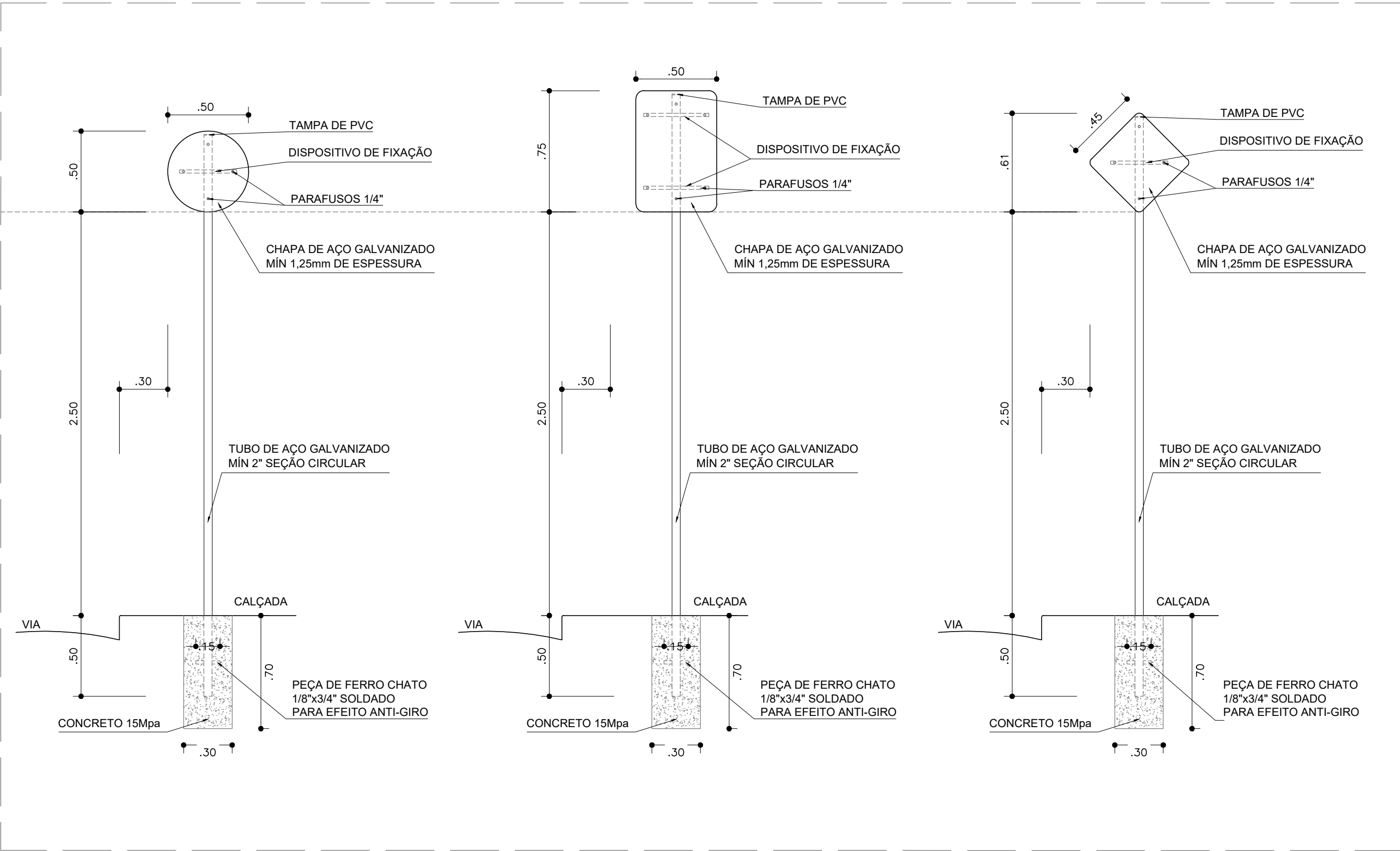
DETALHE 03 – PLACAS DE SINALIZAÇÃO ESCALA 1/20
