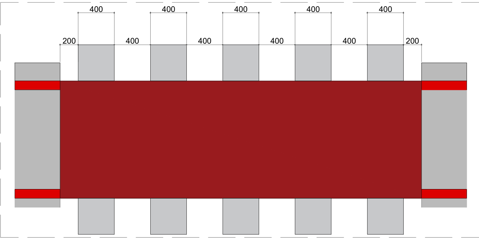
DETALHE 01 – TRAVESSIA CICLOFAIXA ESCALA 1/50
