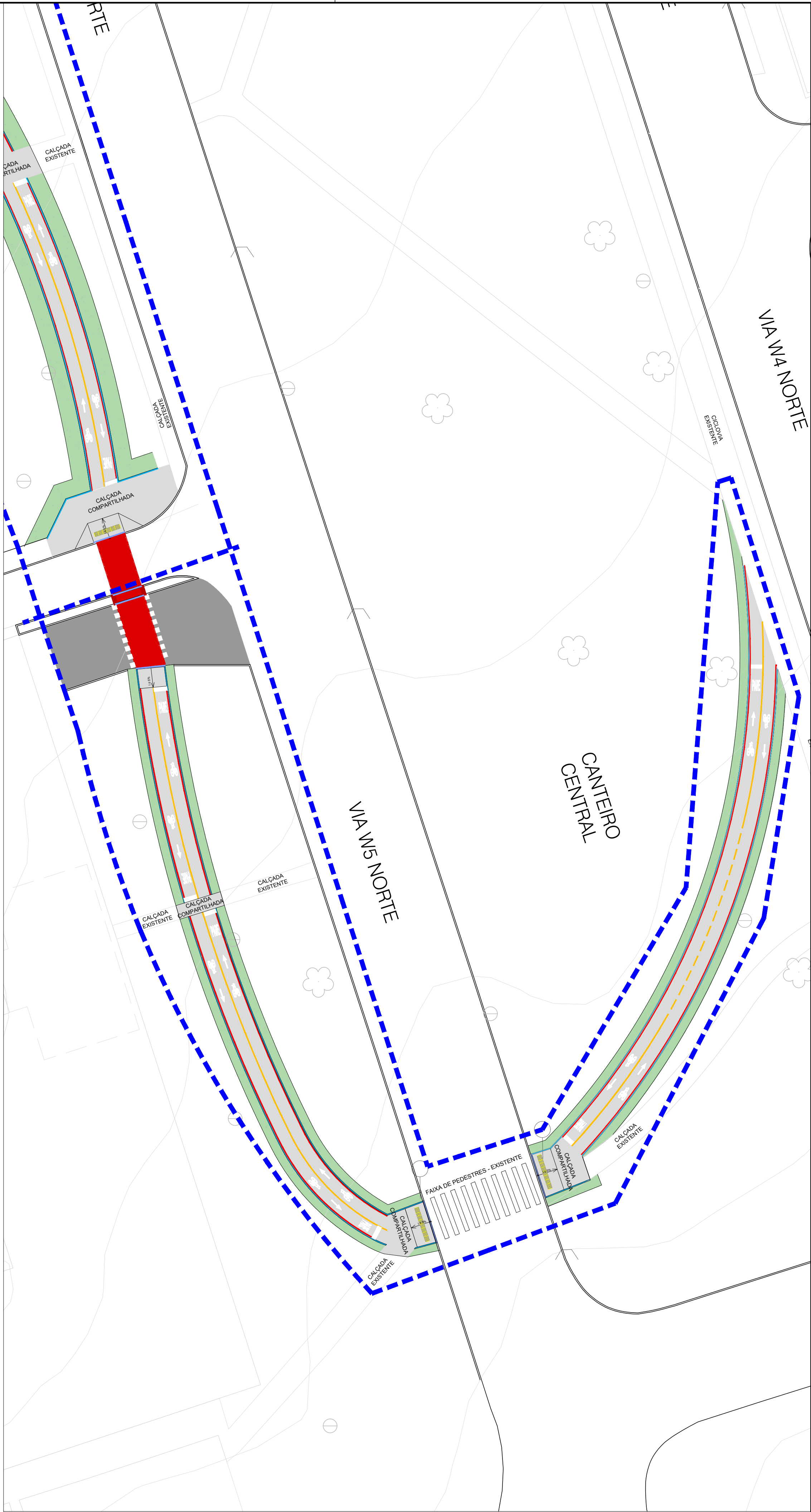
TRECHO 4 ESCALA 1/250
