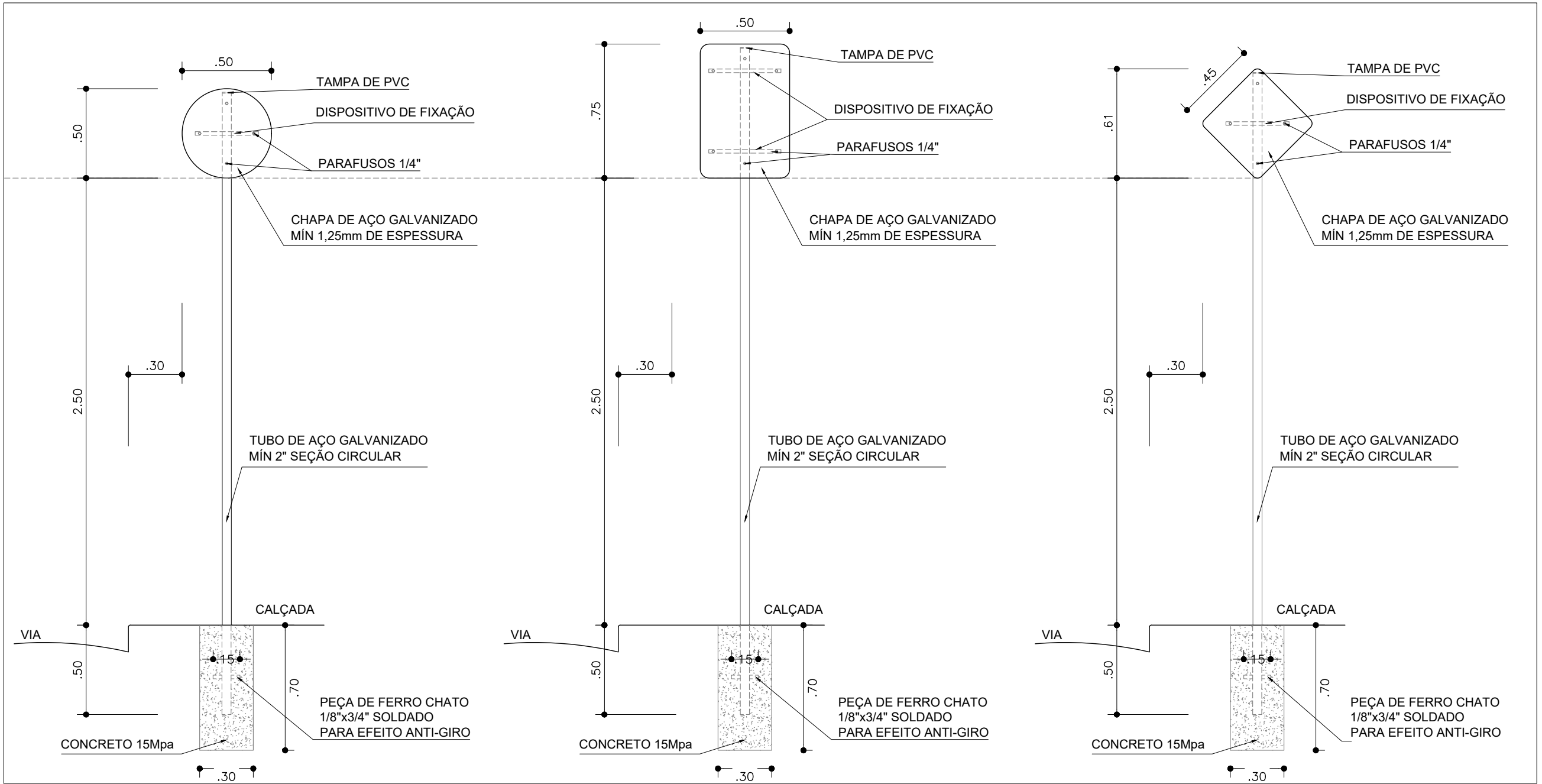
DETALHE 04 ESCALA 1/25
