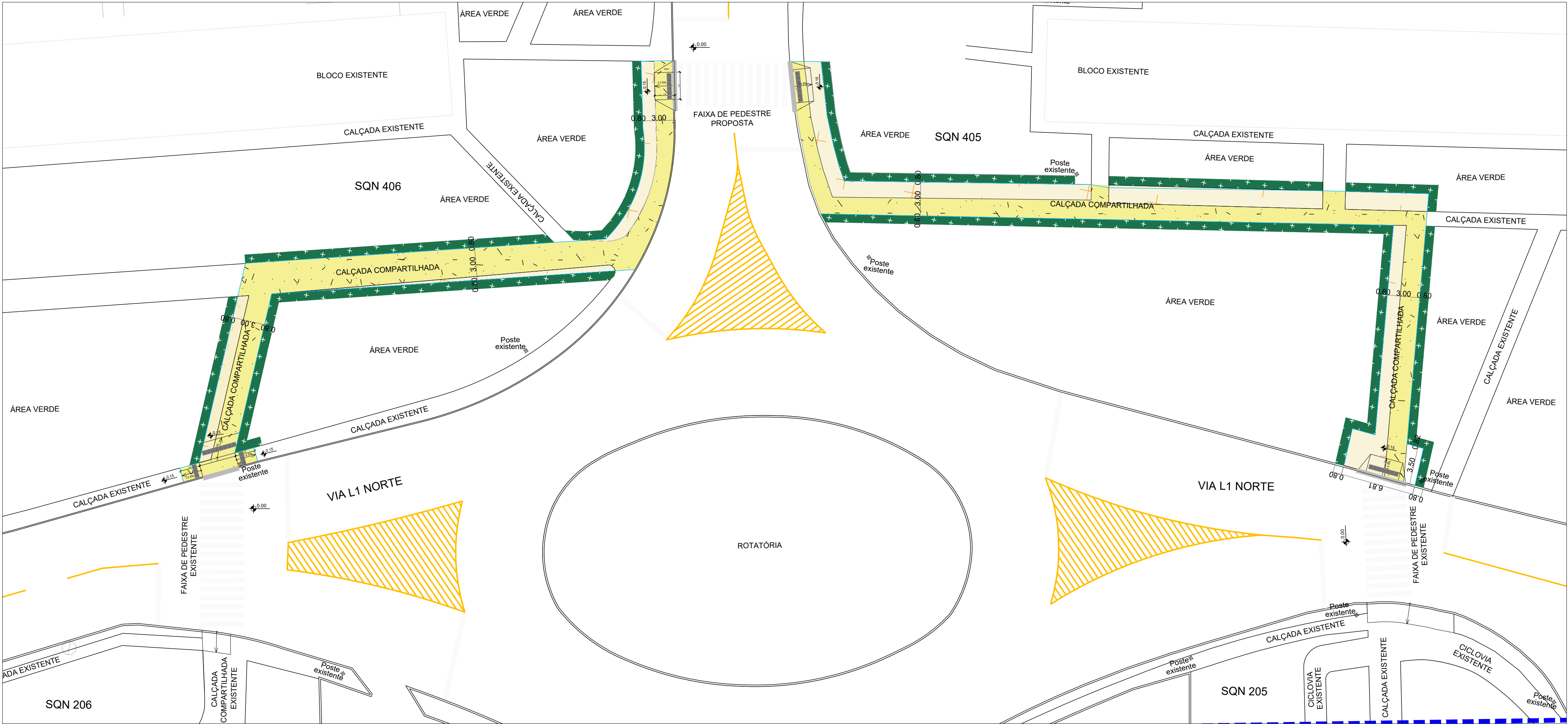
PLANTA – DEMOLIÇÃO ESCALA 1/250
