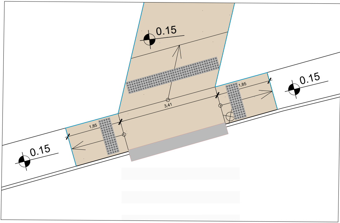
DETALHE 02 ESCALA 1/25
