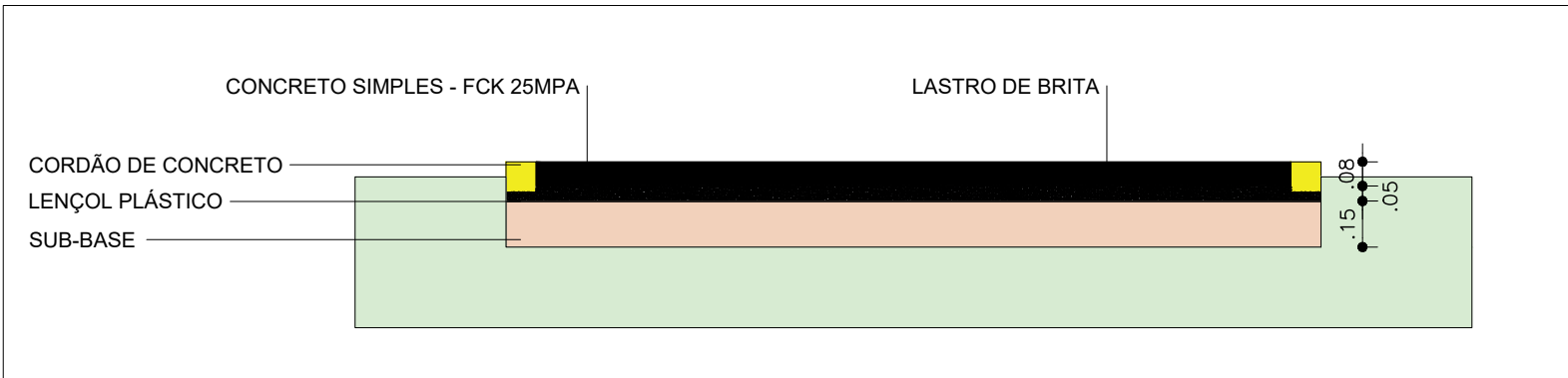
CORTE – PAVIMENTO ESCALA 1/25
