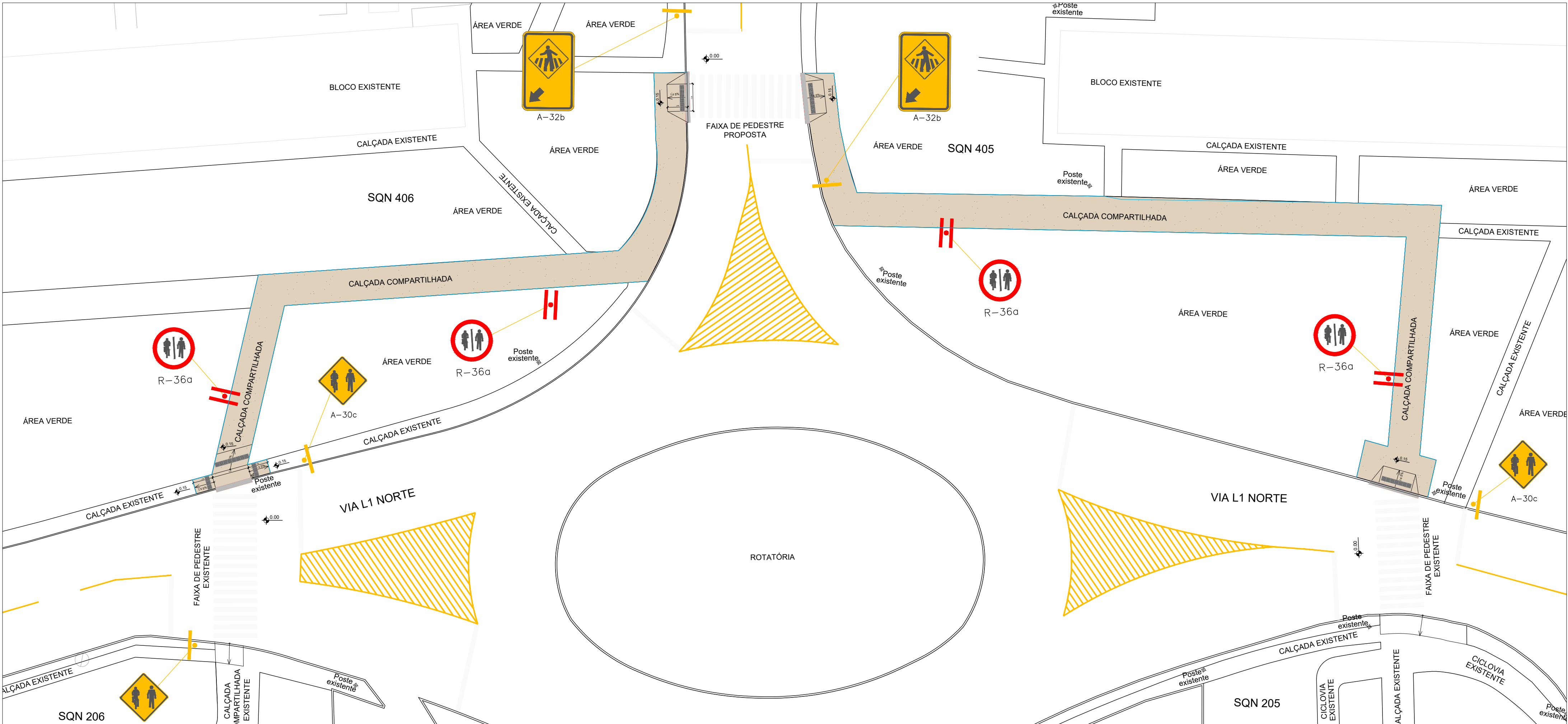
PLANTA – SINALIZAÇÃO ESCALA 1/250
