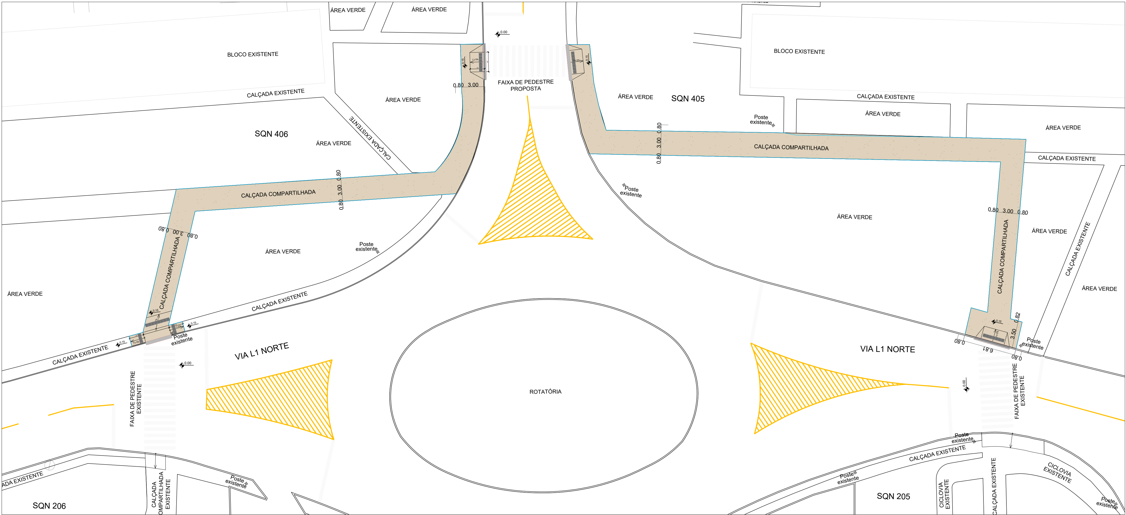
PLANTA – PAVIMENTAÇÃO ESCALA 1/250
